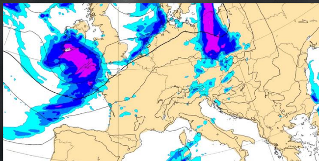
Précipitations
