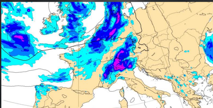
Précipitations
