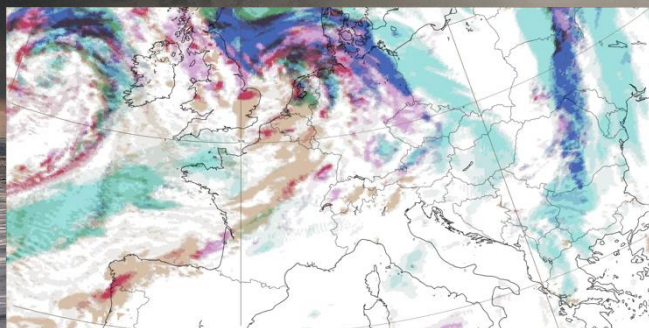
Nébulosité
