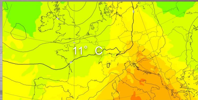
Températures 850 hPa
