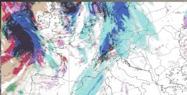
Nébulosité
