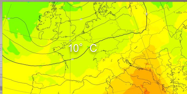
Températures 850 hPa
