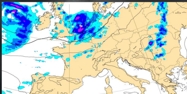
Précipitations
