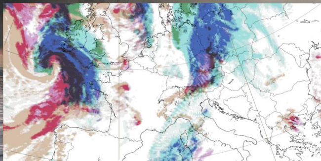
Nébulosité
